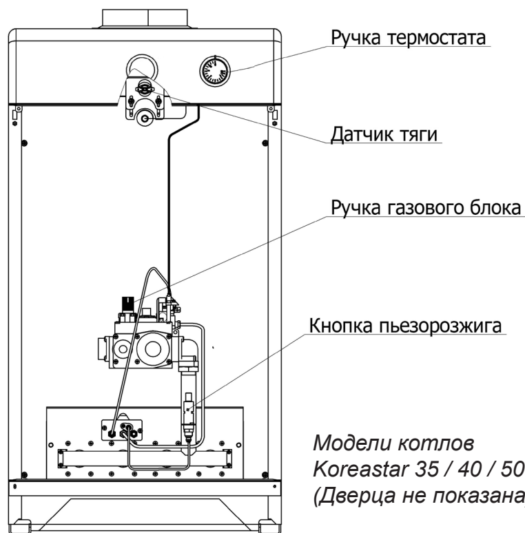
Рисунок 6 - Особенности котлов Koreastar с газовым блоком 820 NOVA MV
