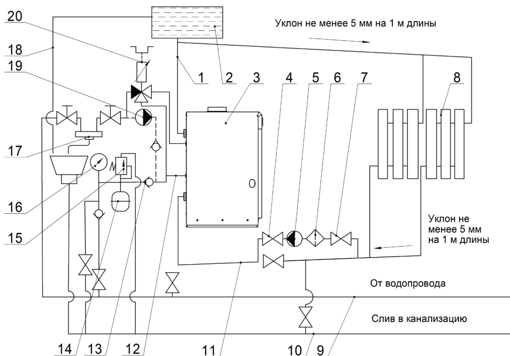
Рисунок 11 - Рекомендуемая гидравлическая схема системы отопления с циркуляционным насосом и схемой автоматического поддержания безопасной температуры (не более 600С) в контуре горячего водоснабжения (ГВС) (С регулятором температуры).
