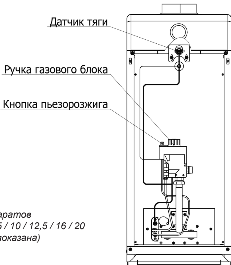
Рисунок 2 - Особенности котлов Koreastar с газовым блоком 630 EUROSIT
