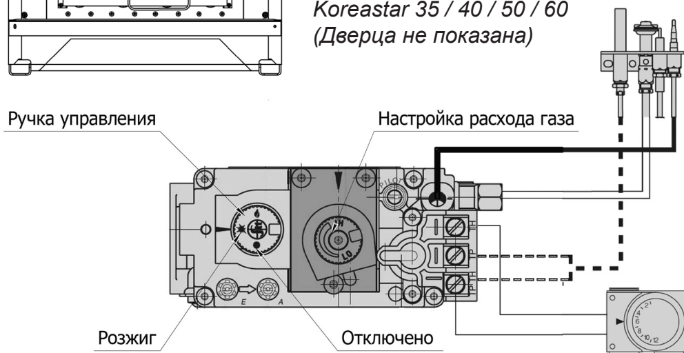
Рисунок 7 - Элементы управления на газовом блоке 820 NOVA MV
