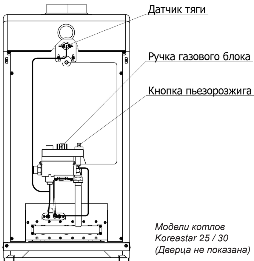
Рисунок 4 - Особенности котлов Koreastar с газовым блоком 710 MINISIT
