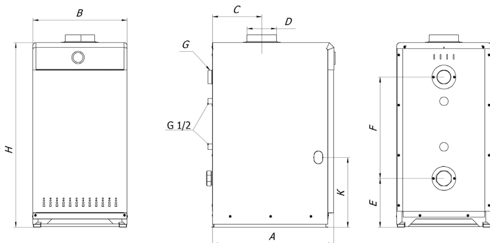
Рисунок 1 - Общий вид, габаритные и присоединительные размеры котлов Koreastar 7,5/ 10/ 12,5/ 16/ 20/ 25/ 30/ 35/ 40 /50 /60
